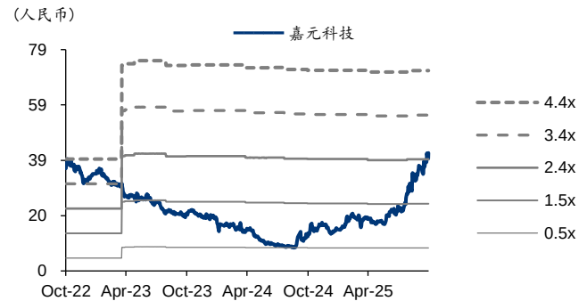
图表3：嘉元科技 PB-Bands
