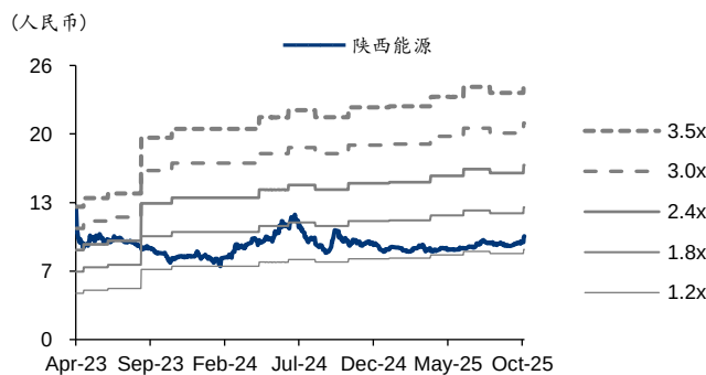
图表5：陕西能源 PB-Bands
