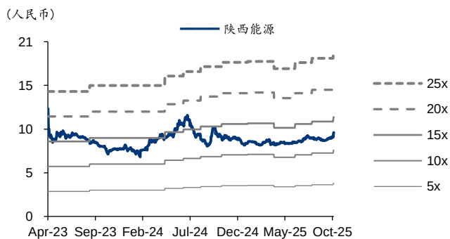
图表4：陕西能源 PE-Bands
