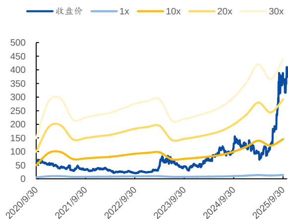
图 2: P/B Band
