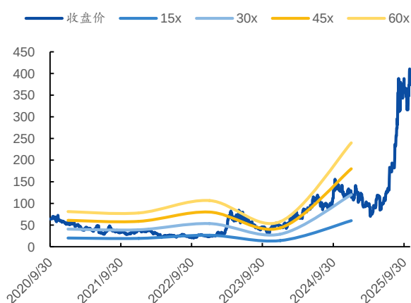
图 1: P/E Band
