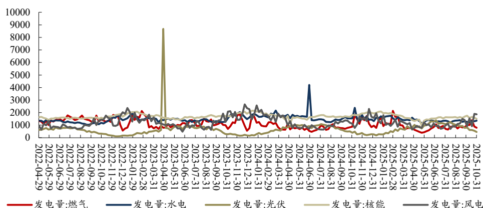
图7：最近一年欧洲发电结构（GWh/日，周度数据，截至 2025/10/31）
