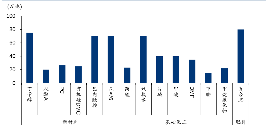
图表2：鲁西化工代表性产品产能布局情况（截至 2025 年 10 月）
