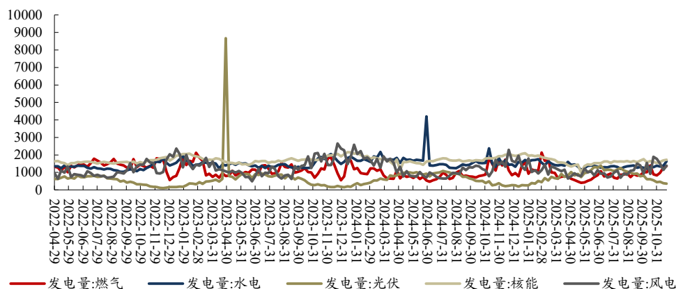
图7: 最近一年欧洲发电结构 (GWh/日, 周度数据, 截至 2025/11/21)
