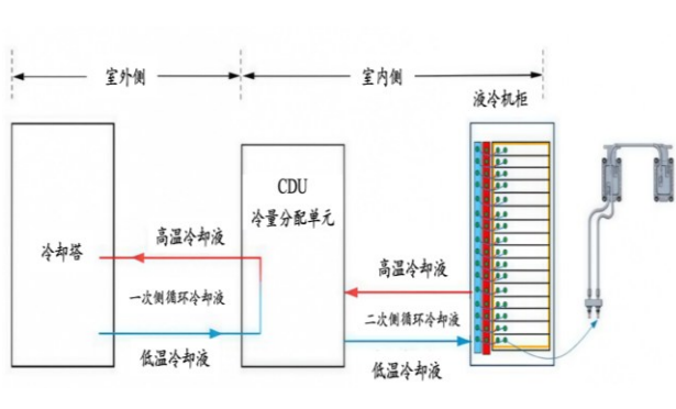
图28：冷板式液冷系统原理图
