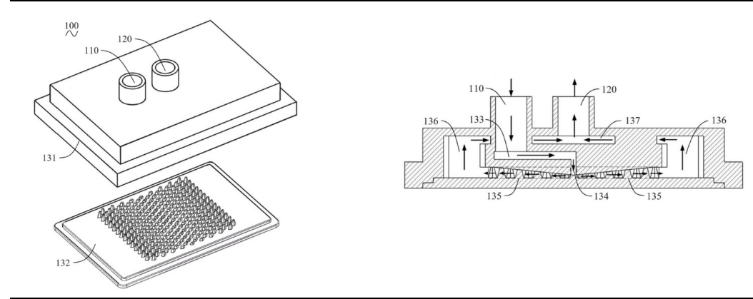
图36：英维克“微通道冷板”实用新型专利示意图
