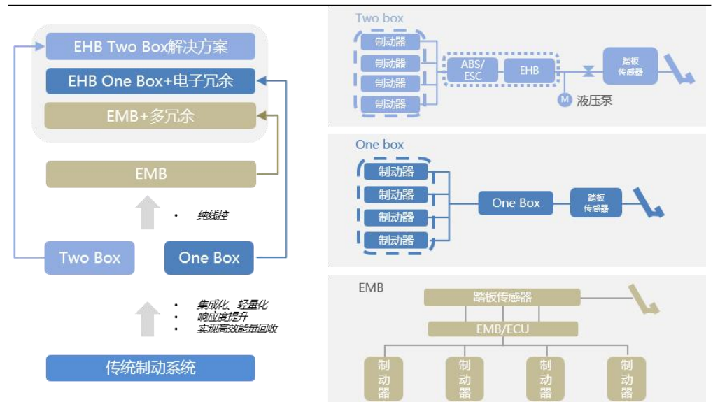
图表 32：线控制动三种方案的系统架构
