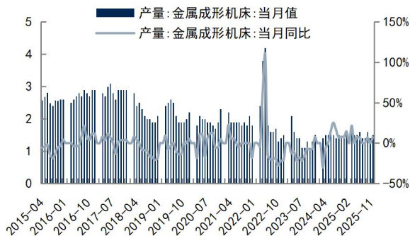
图20: 2025 年 11 月金属成形机床产量同比增长 7.10%
