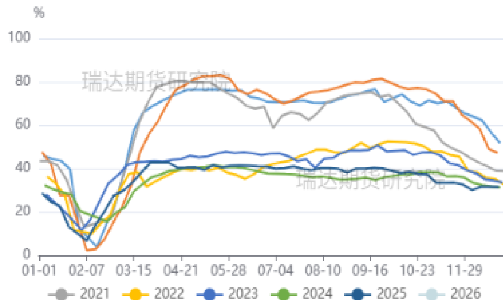
图14、水泥发运率
