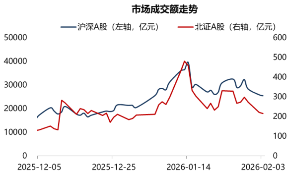
图1: 市场成交额走势 (截至 2026/2/3)
