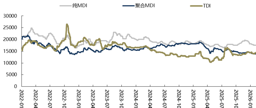
中国纯MDI、聚合MDI、TDI价格走势（元/吨）
