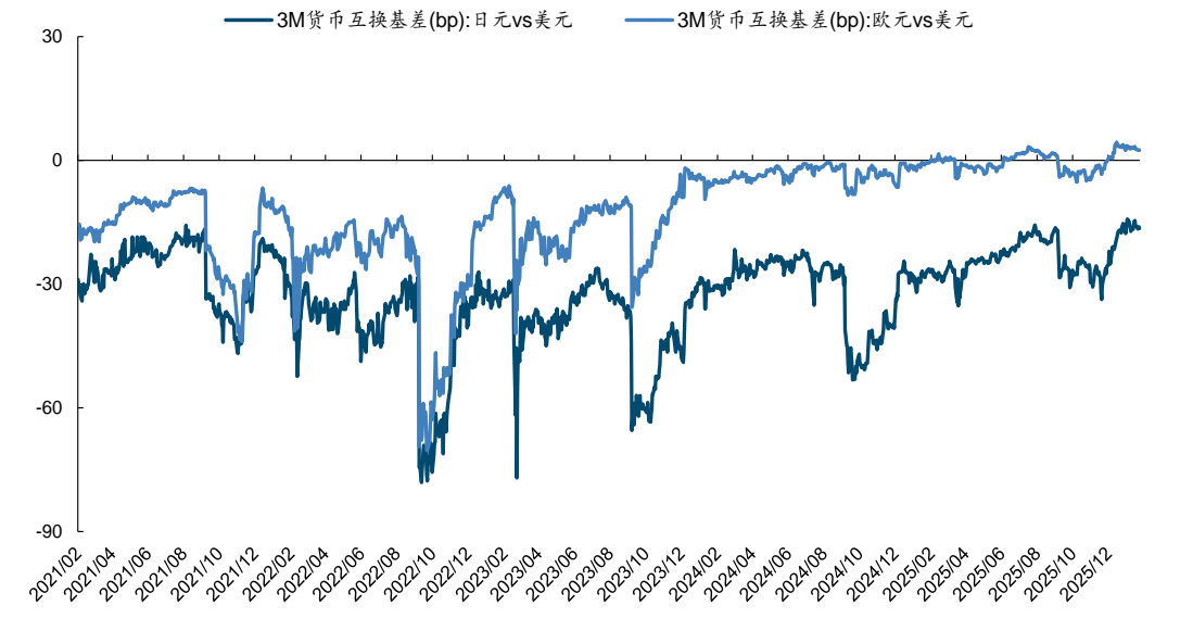
图表5: 春节前一周3个月日元/欧元与美元互换基差均回落
