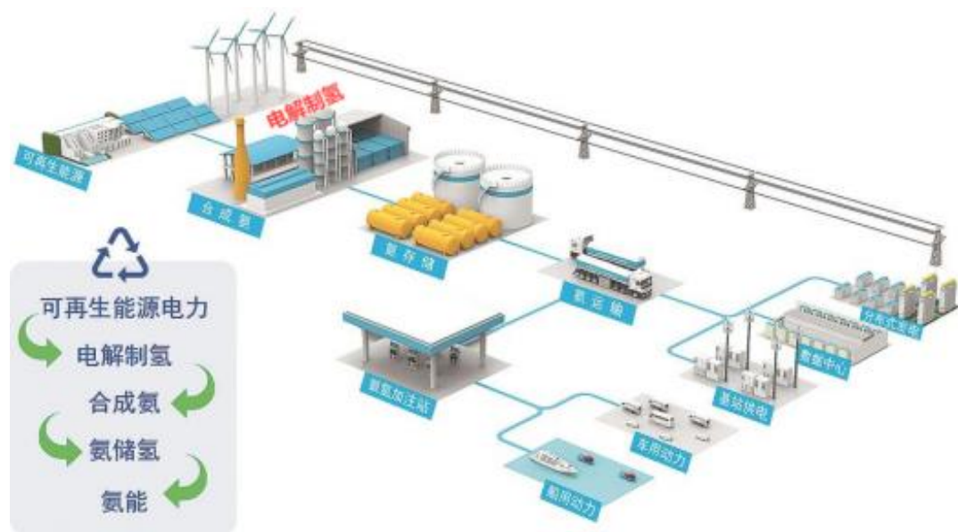
图4：绿色“氨-氢”能源“零碳”循环路线
