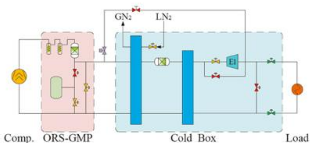
10kW@20K氮制冷机
