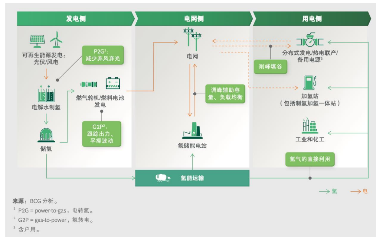
图 2：氢储能在可再生能源电网中的应用
