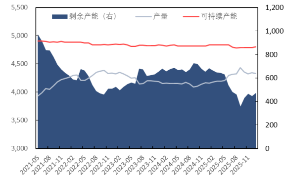
图 37: OPEC+ 产能、产量及剩余产能 (万桶/日, 万桶/日)
