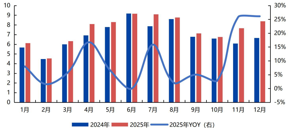
图表 12: 国内逆变器月度出口金额 (亿美元、%)
