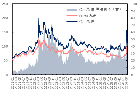
图 47：原油、欧洲柴油价格及价差（美元/桶，美元/桶）
