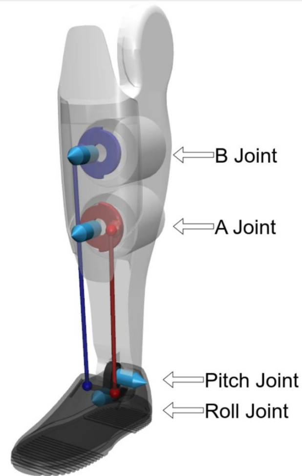
图表41：小腿连杆示意图
