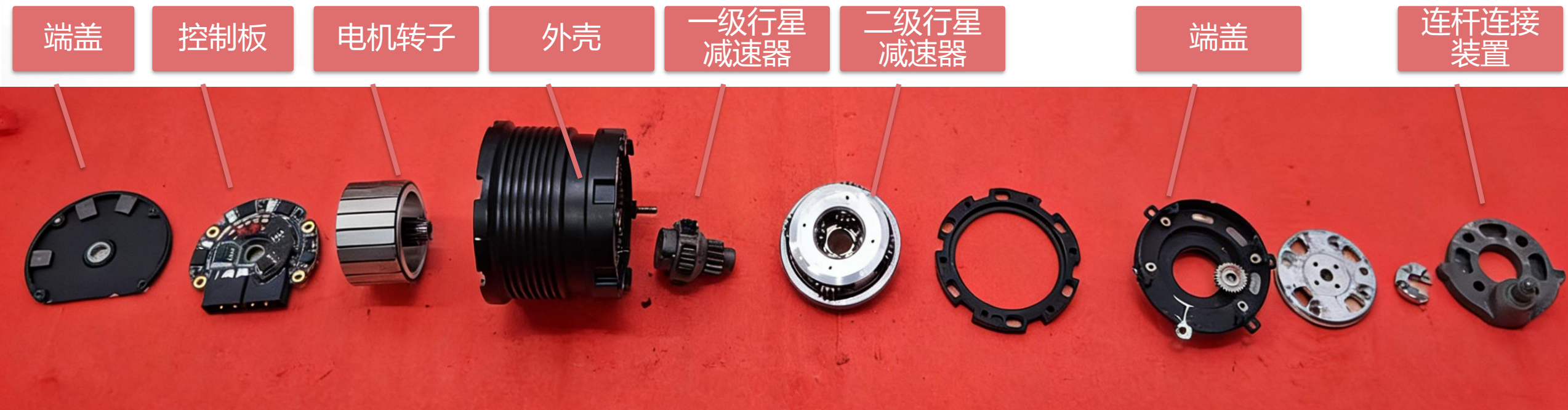
图表13：小腿处小关节爆炸图
