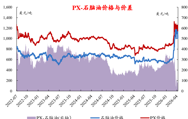
图19：本周PX-石脑油价差扩大
