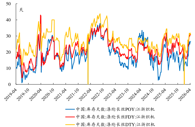
图6：本周涤纶长丝 POY 库存天数小幅上涨
