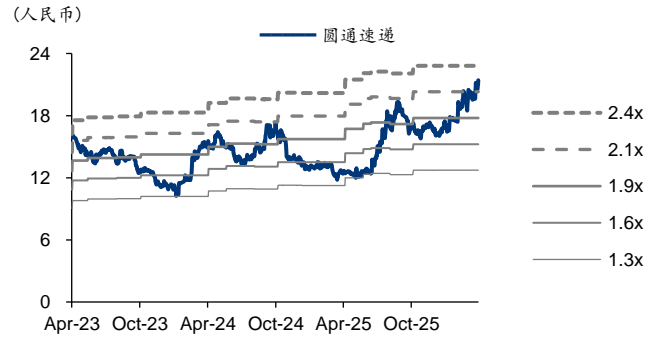
图表5: 圆通速递 PB-Bands
