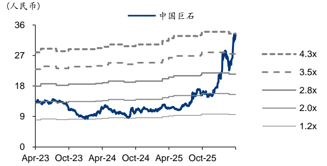
图表3: 中国巨石 PB-Bands
