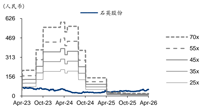
图表2: 石英股份 PE-Bands
