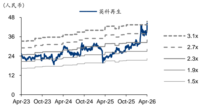
图表5: 英科再生 PB-Bands
