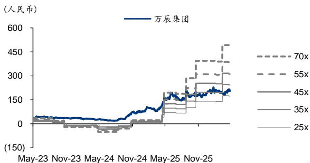
图表2：万辰集团 PE-Bands
