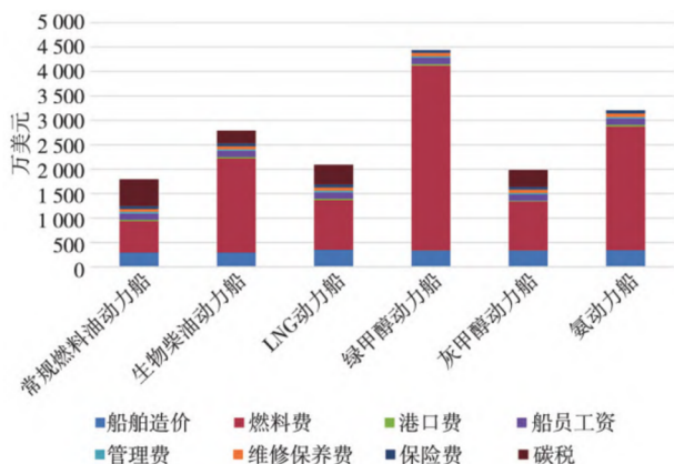
图表34：不同动力船成本预估
