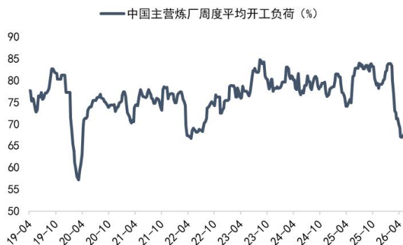
图25: 中国主营炼厂周度平均开工负荷 (%)
