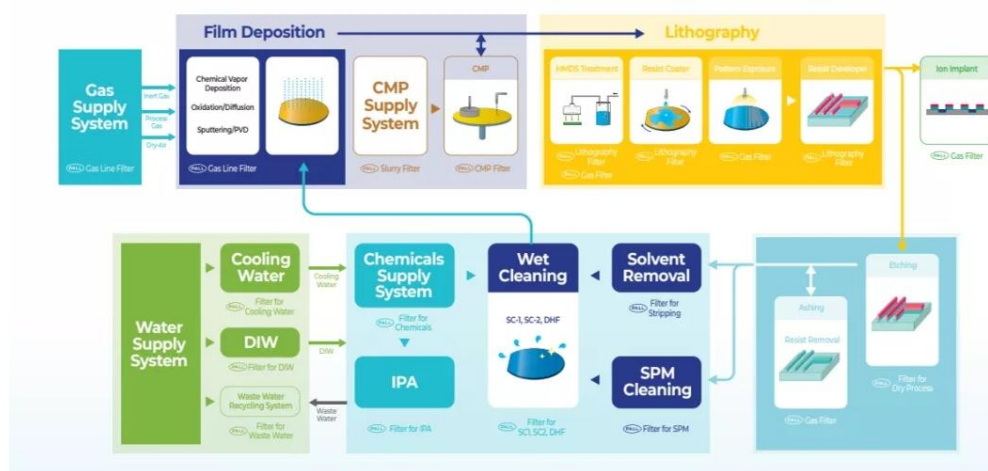
图表 3：晶圆加工流程涉及过滤步骤
