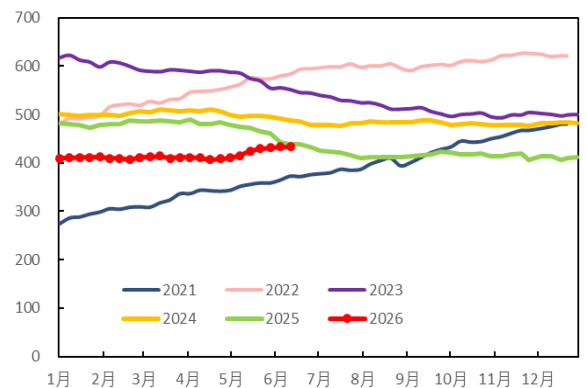
图 15：美国原油钻机数（台）
