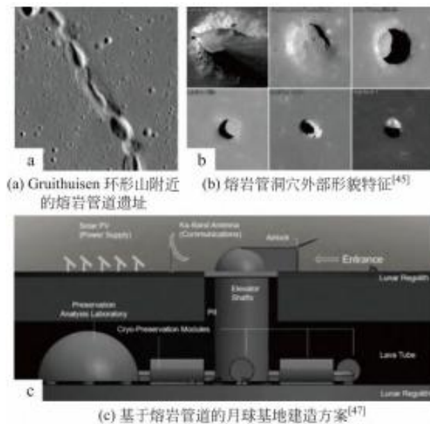
图：月球熔岩管道地下结构示意图
