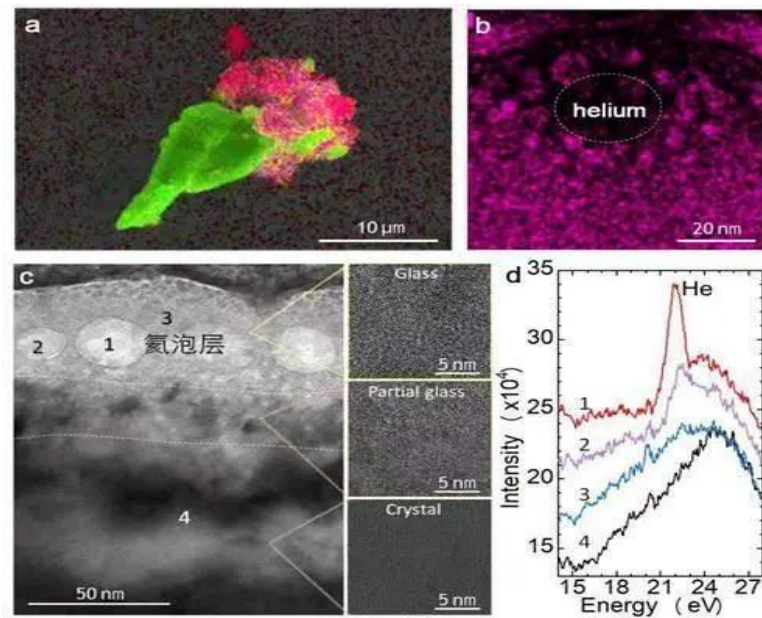
图：月壤中发现的氦-3资源
