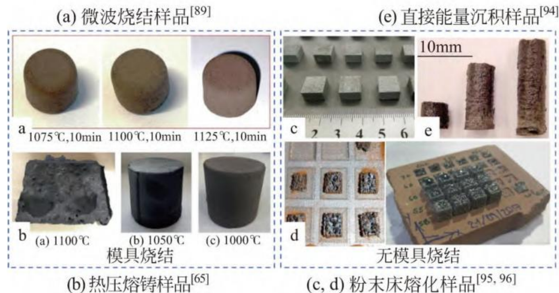
图：烧结类星壤材料
