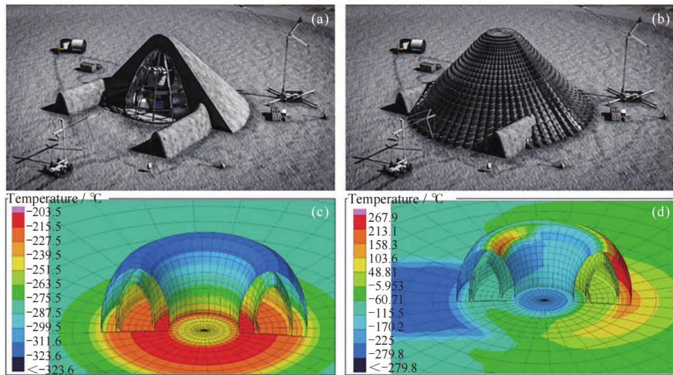
图 5 月球庇护所。(a) 概念, (b) 支撑结构, (c) 夜晚结构热分析, (d) 月午结构热分析
