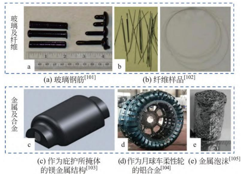
图：星壤衍生材料
