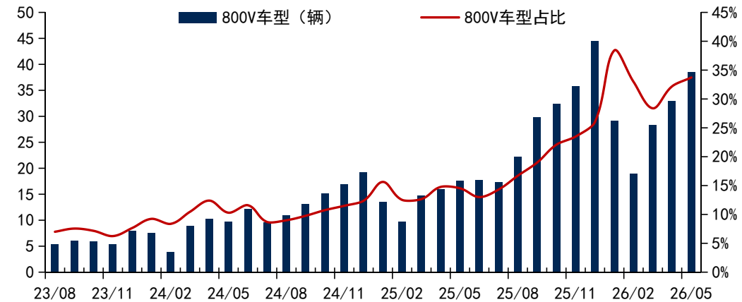
图：23-26年我国新能源上险乘用车中800V车型占比（%）
