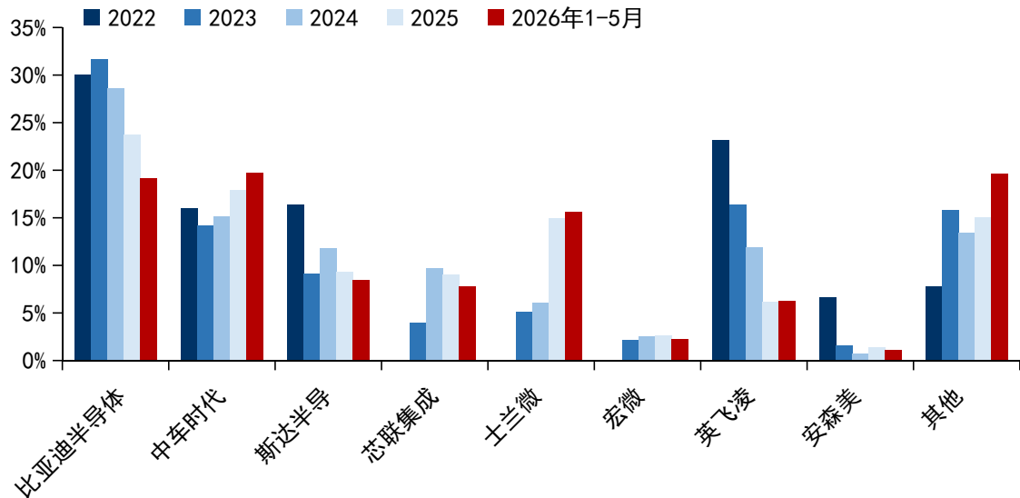
图：22-26年我国新能源上险乘用车主驱IGBT模块电控搭载量分布（按厂商，%）
