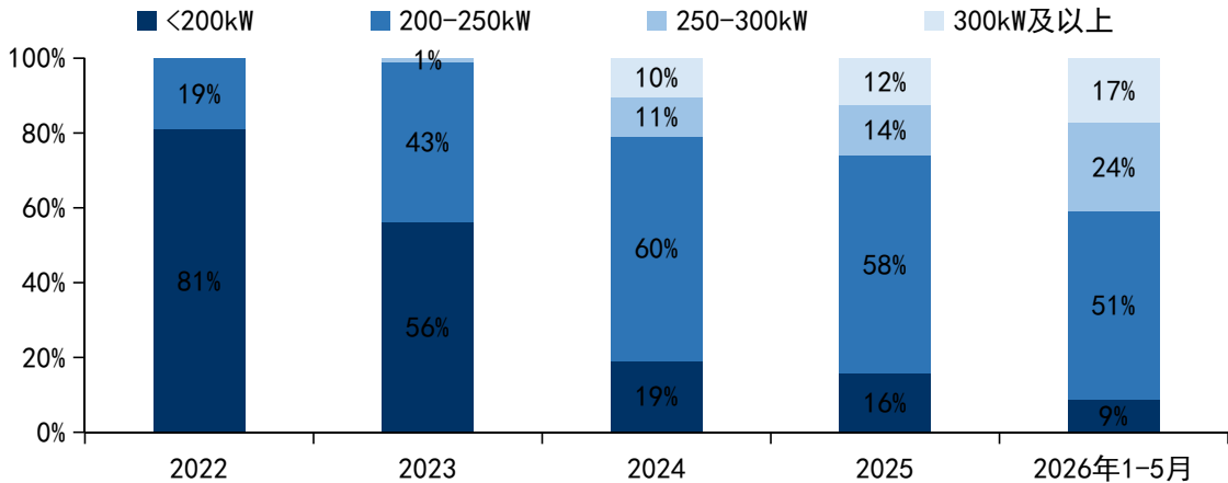
图：22-26年我国新能源上险乘用车碳化硅电控功率段分布（%）
