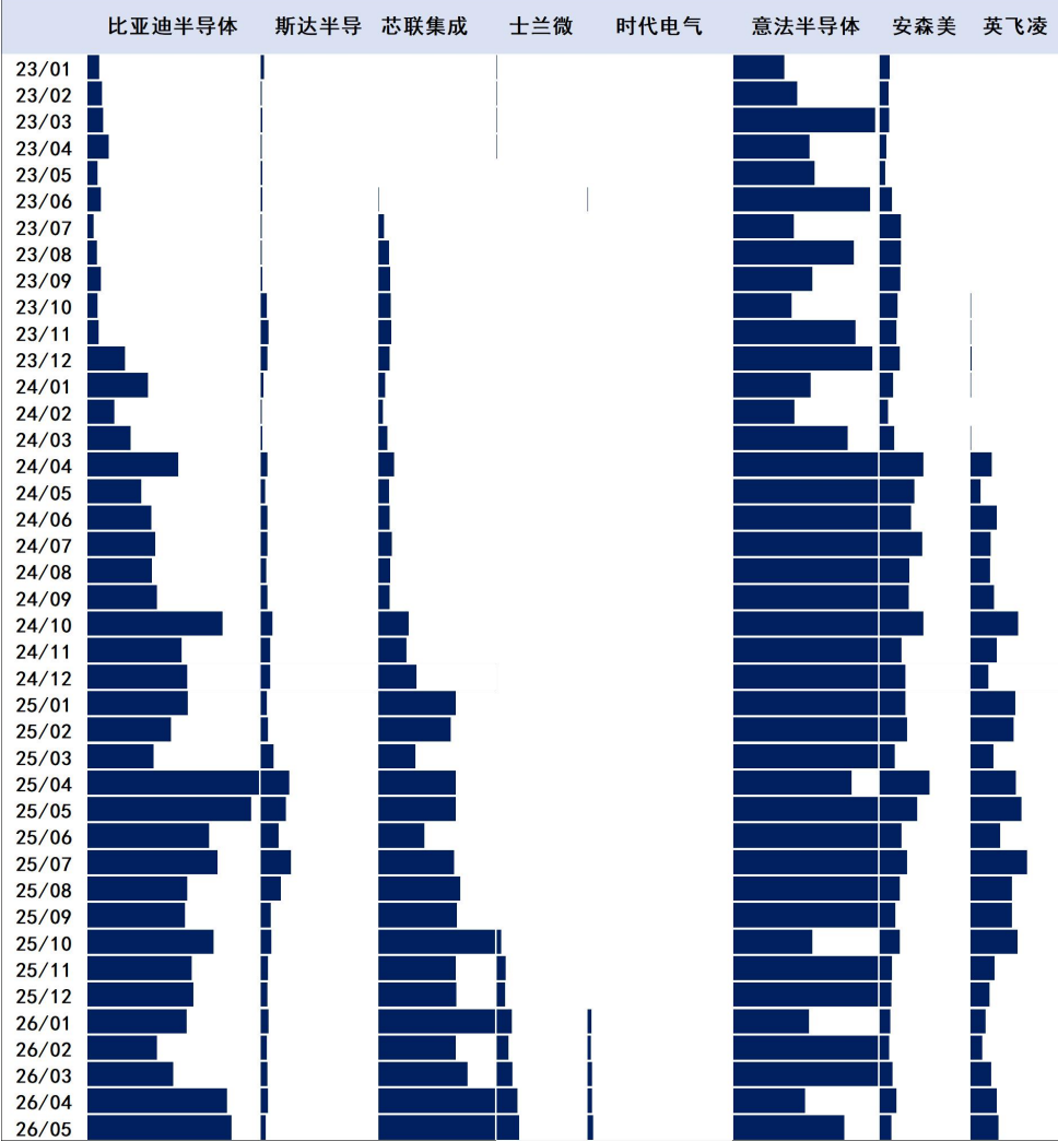
图：22-26年我国新能源上险乘用车SiC功率模块代表厂商出货量
