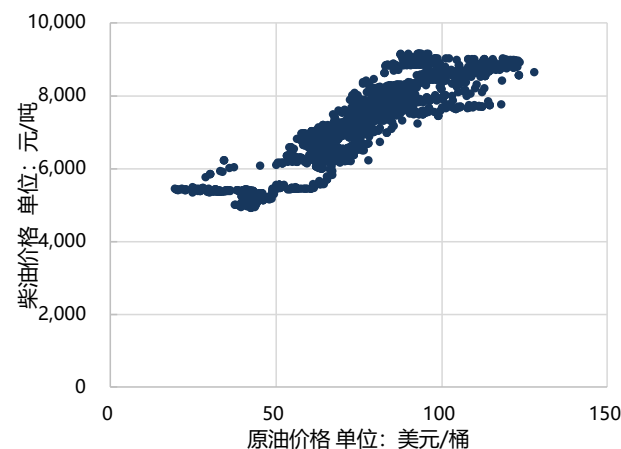
2017-2026年6月国际原油价格与国内柴油价差（元/吨，美元/桶）
