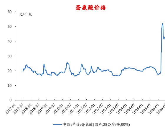
图61：本周蛋氨酸价格下跌
