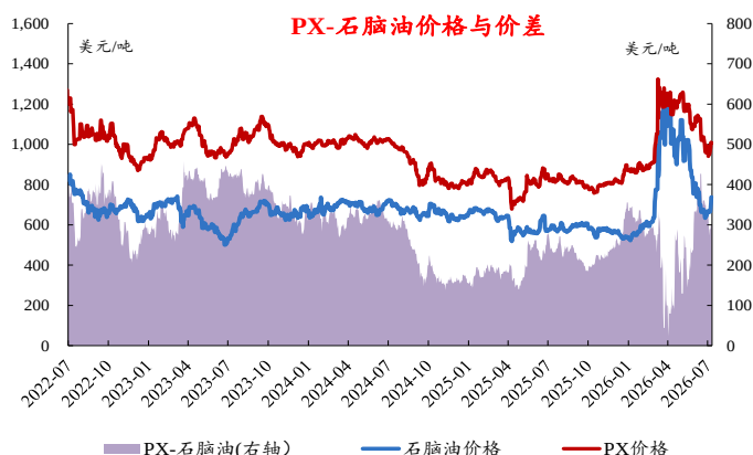
图21: 本周PX-石脑油价差收窄
