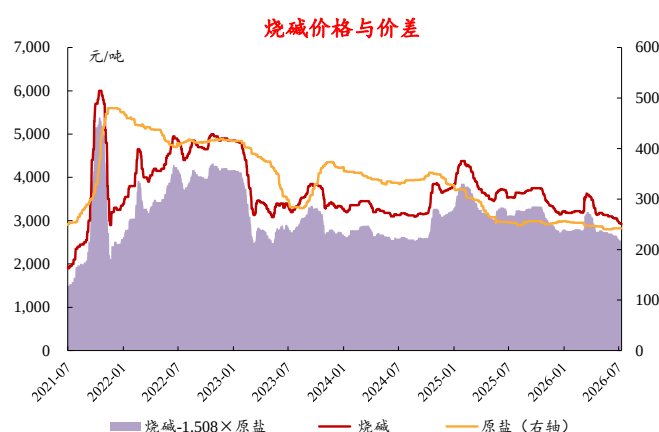
图45：本周烧碱价差收窄
