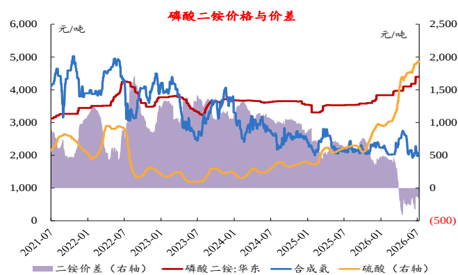
图51: 本周磷酸二铵价差为负
