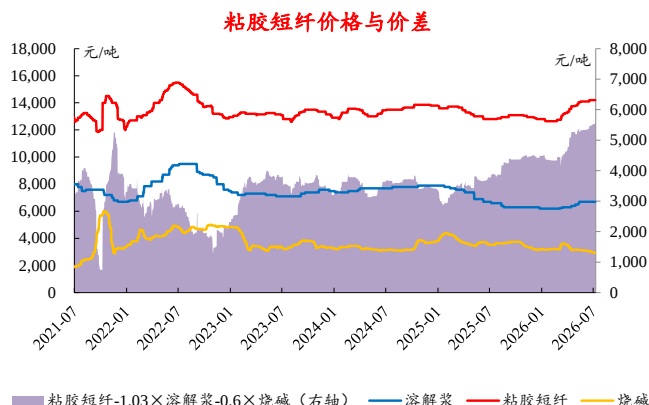
图10：本周粘胶短纤价差小幅扩大
