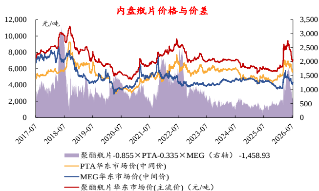
图30: 本周聚酯瓶片价差收窄
