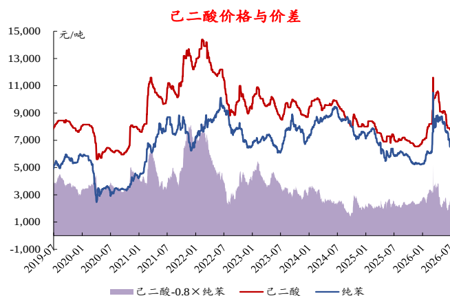
图27: 本周己二酸价差收窄
