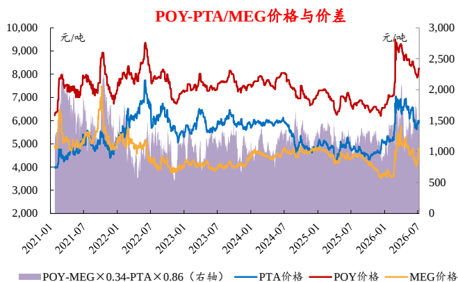
图24: 本周POY-PTA/MEG 价差扩大
