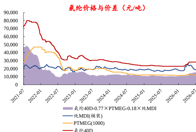
图12：本周氨纶价差小幅收窄
