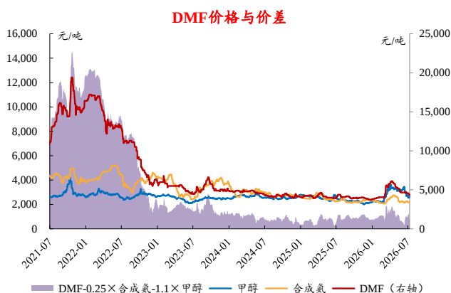
图40：本周DMF价差扩大
