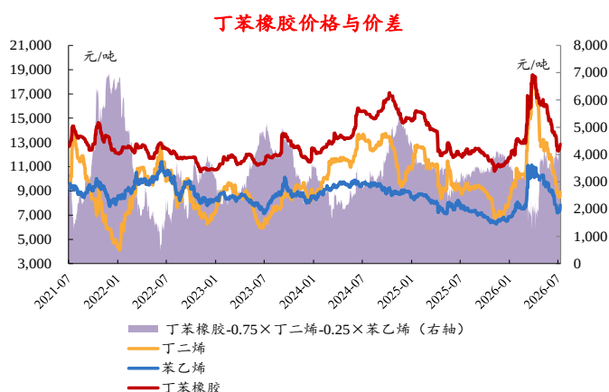
图29: 本周丁苯橡胶价差收窄
