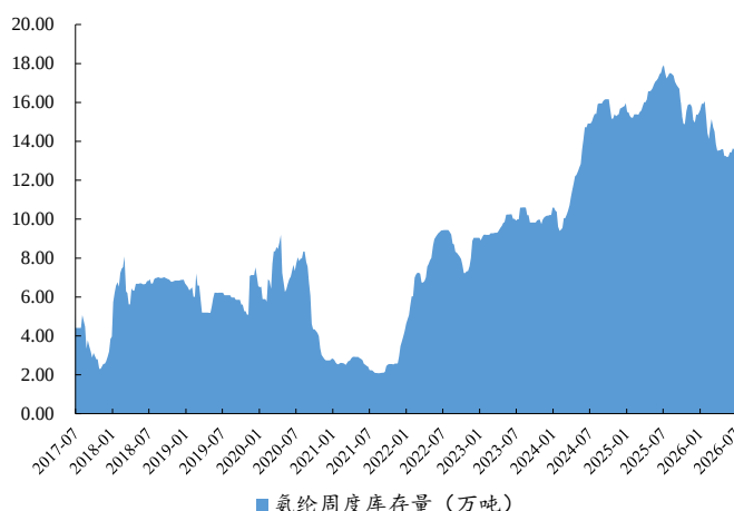
图13：本周氨纶库存小幅增加
