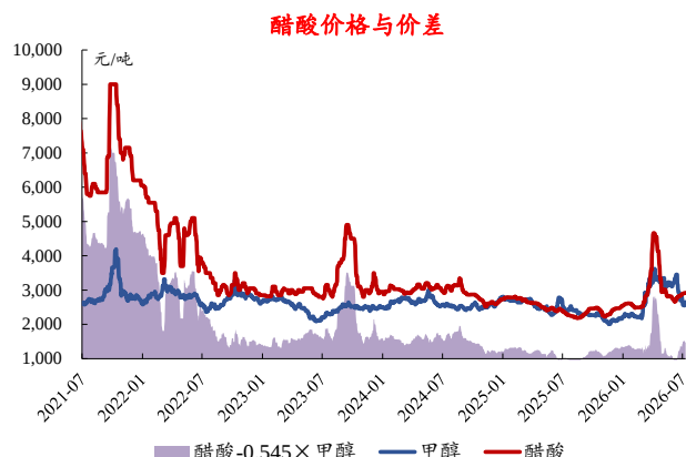
图41：本周醋酸价差扩大
