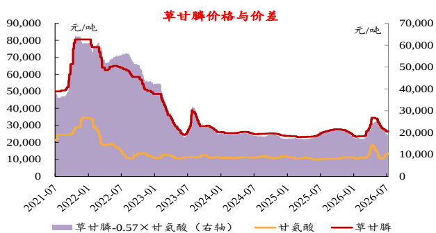
图52: 本周草甘膦价差收窄
