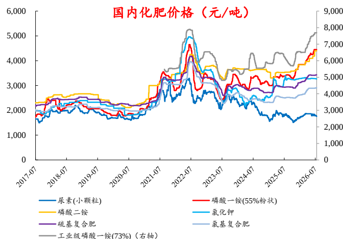
图16：本周国内尿素价格小幅下降
