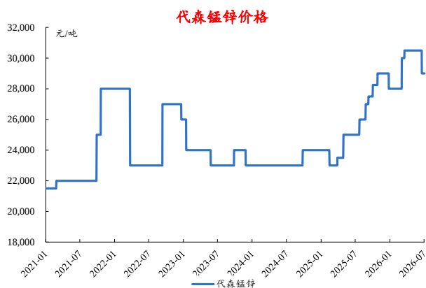
图54: 本周代森锰锌价格稳定
