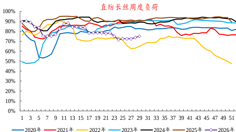
图5：截至本周五，涤纶长丝行业负荷为 75.1%
