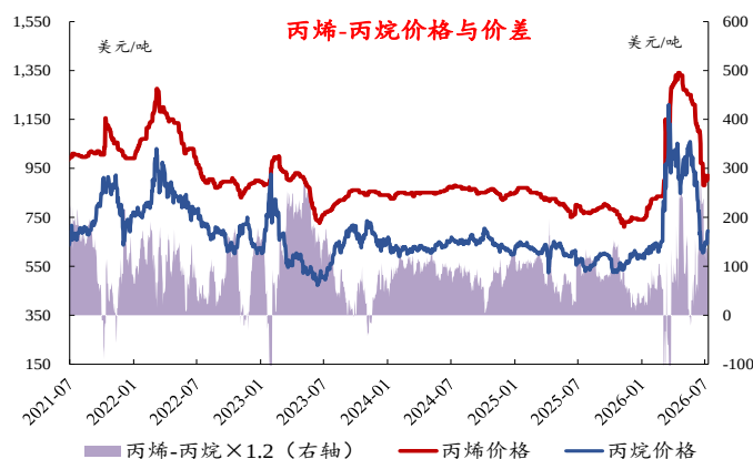
图23: 本周丙烯-丙烷价差收窄
