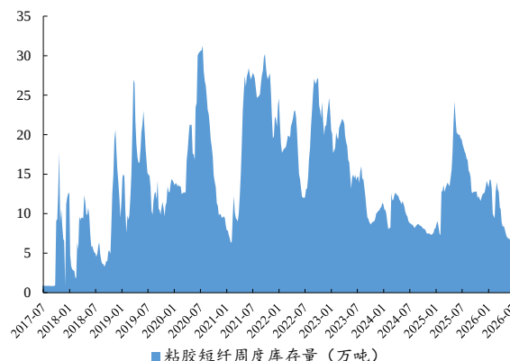
图11：本周粘胶短纤库存小幅上升
