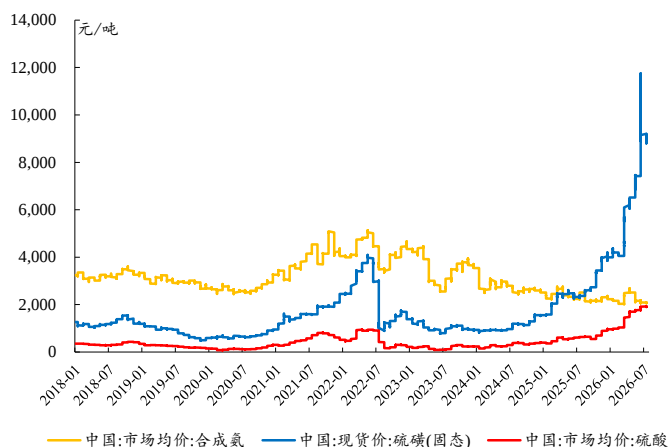
图14：本周硫酸价格小幅下降
