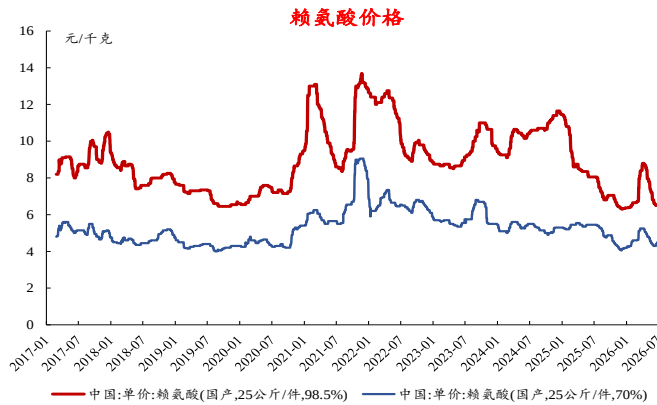
图62：本周赖氨酸（98.5%）价格基本稳定
