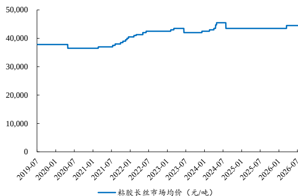
图35：本周粘胶长丝市场均价基本稳定
