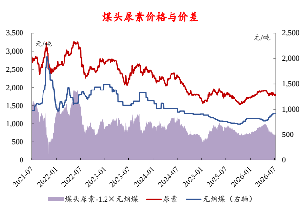
图39：本周煤头尿素价差稳定
