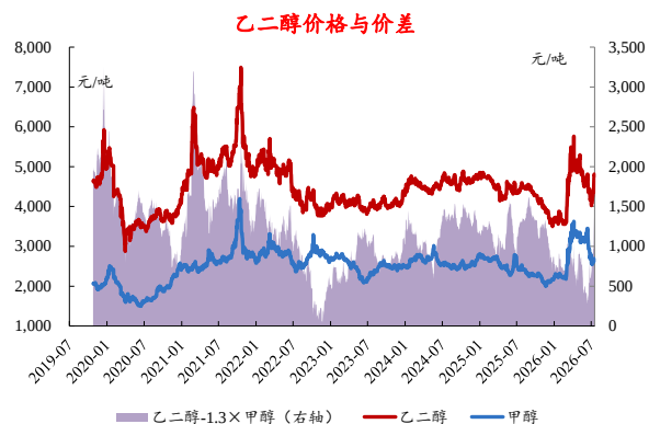
图43：本周乙二醇价差扩大
