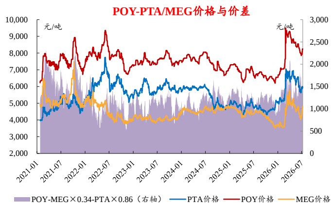
图33：本周 POY-PTA/MEG 价差扩大
