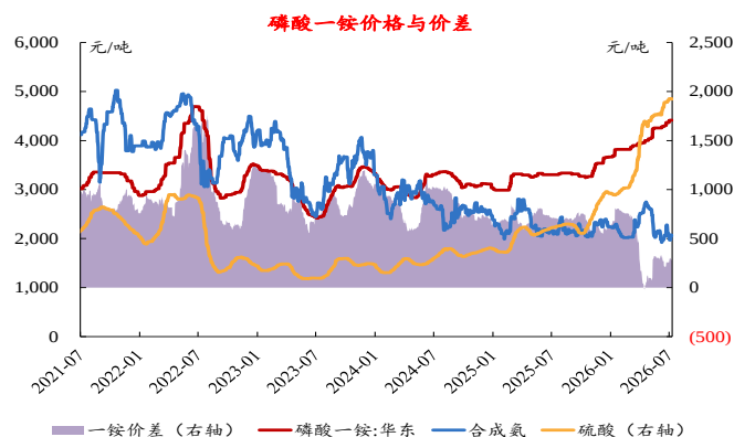
图50: 本周磷酸一铵价差扩大
