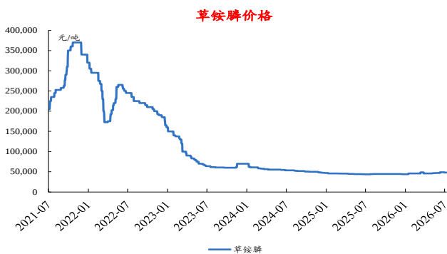
图53: 本周草铵膦价格稳定
