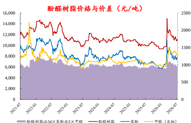
图31: 本周酚醛树脂价差扩大
