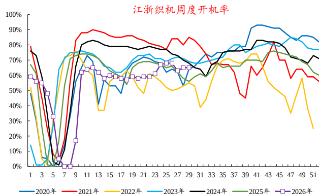
图7：截至本周五，涤纶长丝下游织造开机率为 65%
