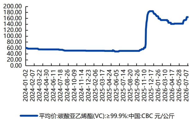
图表 5：碳酸亚乙烯酯平均价
