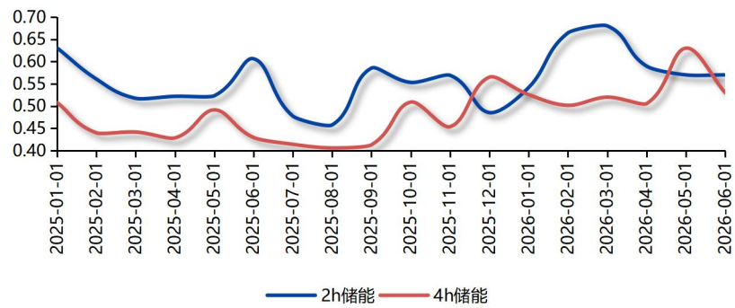
图表 7：国内储能系统月度中标加权均价（元/Wh）
