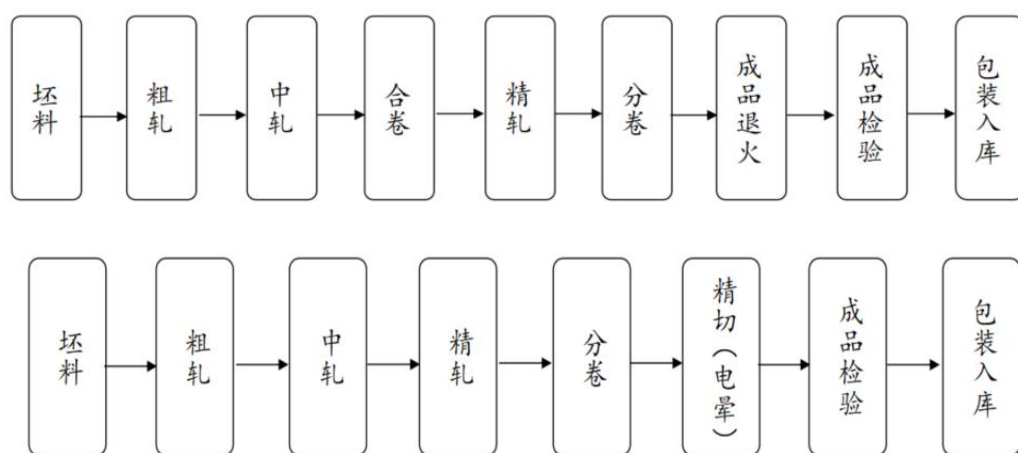
图表5：公司电池铝箔和包装箔工艺流程
