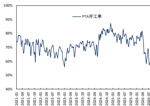
图 67: PTA 开工率 (%)
