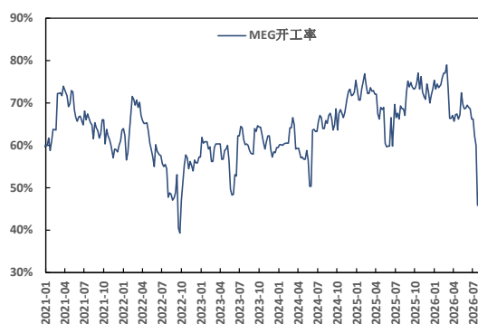
图 61: MEG 开工率 (%)
