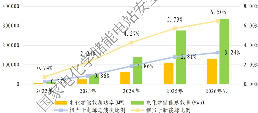
图 1-1 电化学储能近 5 年发展情况
