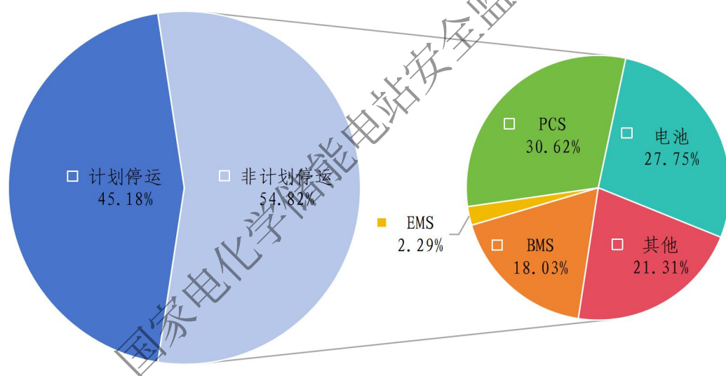
图 4-1 2026 年上半年电化学储能停运次数分布情况
