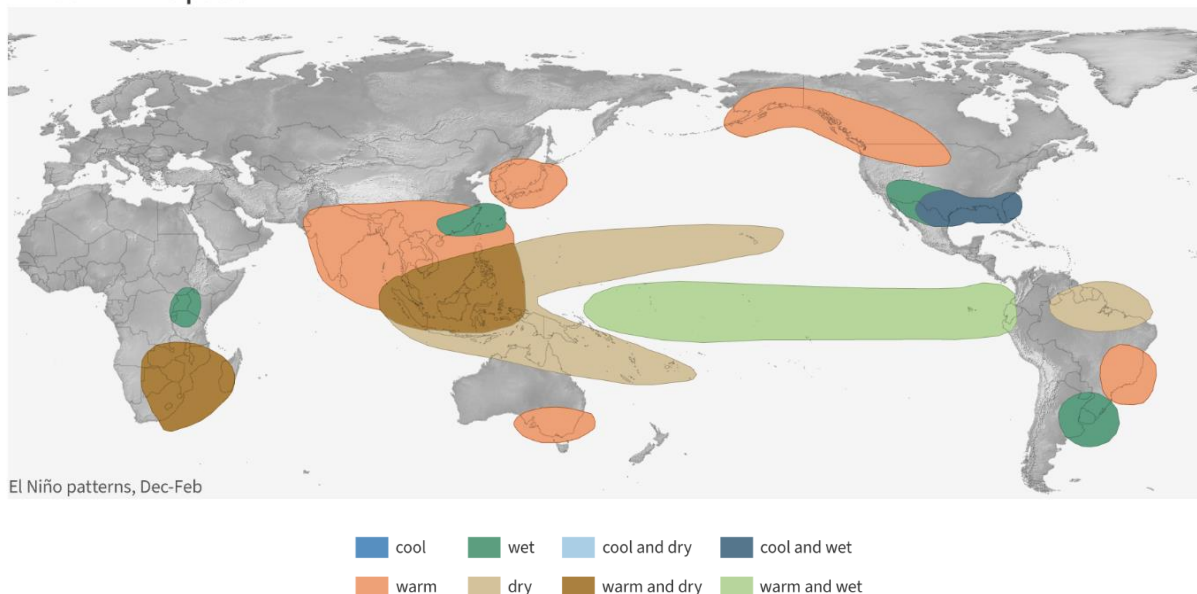
Winter El Niño pattern
