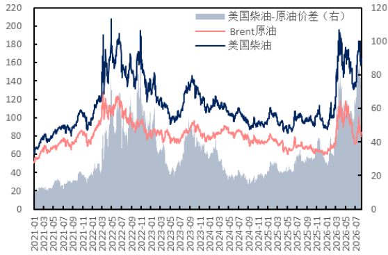
图 45：原油、美国柴油价格及价差（美元/桶，美元/桶）
