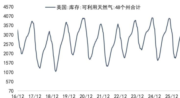
图64: 美国天然气库存量（十亿立方英尺）
