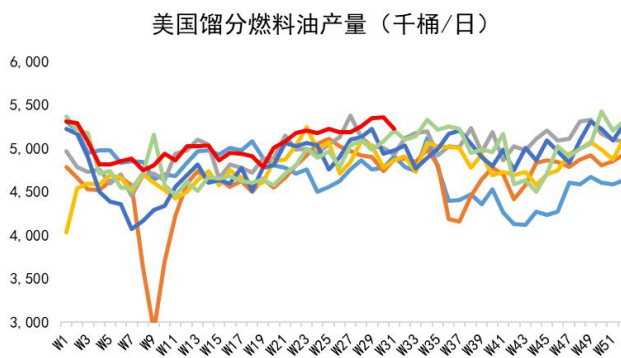
图46: 美国柴油产量（千桶/天）
