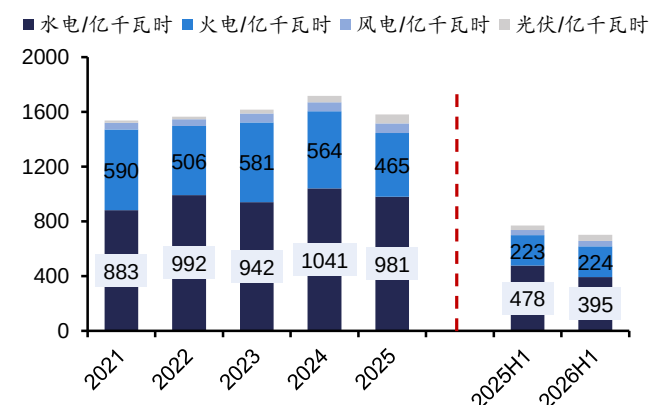
图表6: 近年公司各电源发电量
