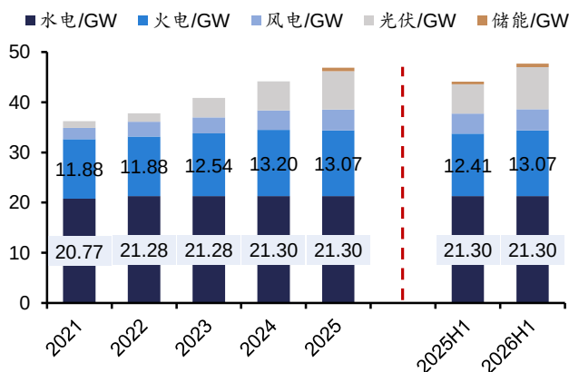
图表5: 截至 2026H1 公司总装机 47.7GW
