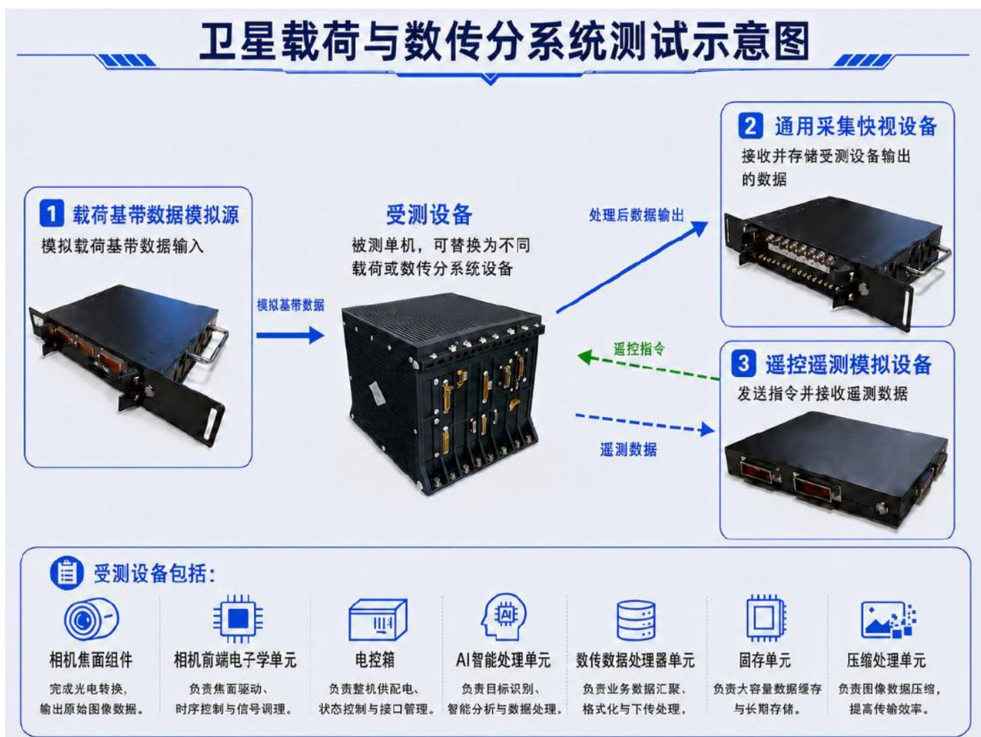
图1：卓目科技光学遥感卫星载荷与数传分系统测试产品示意图
