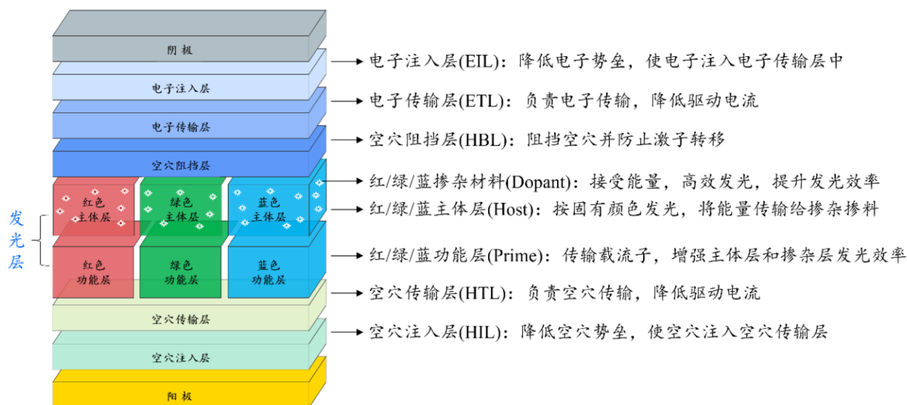
图9: AMOLED 多层有机薄膜的器件结构
