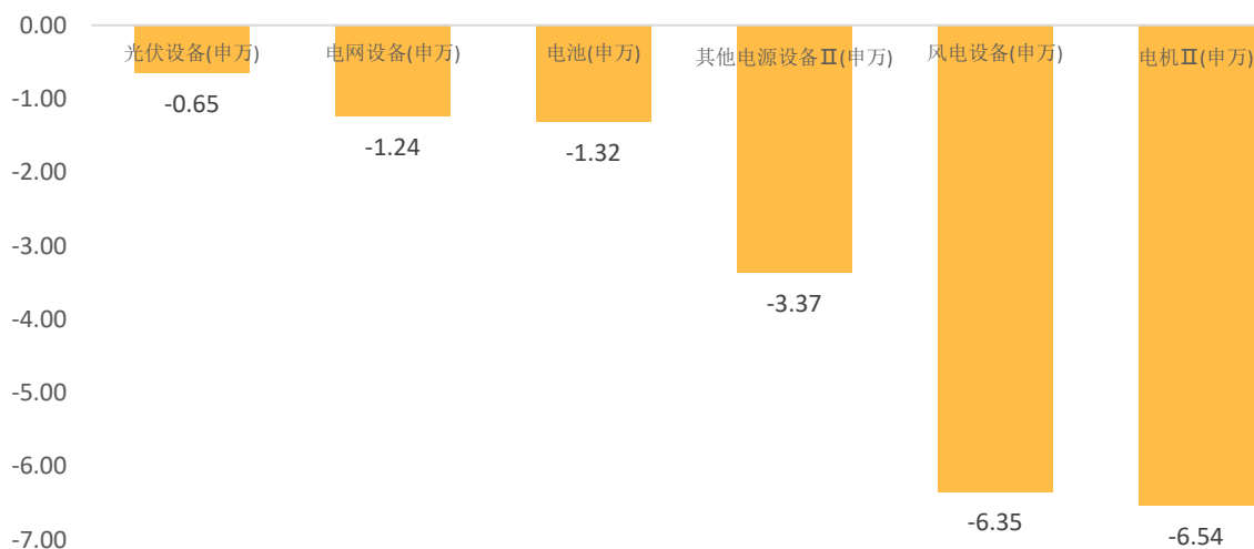
图表 2：本周光伏设备（申万）行业指数-0.65%（%）
