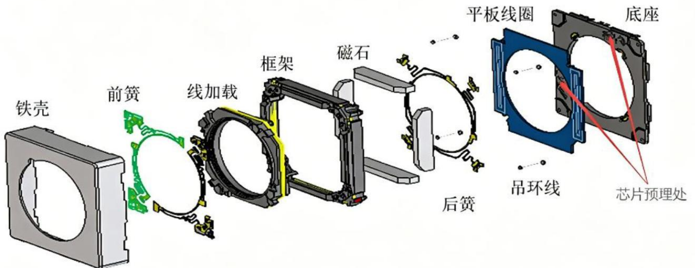
图10：摄像头马达结构示意图
