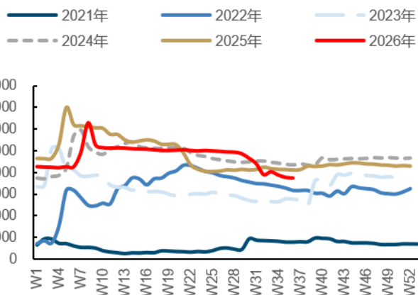
图表21: 铜铁库存 (吨)
