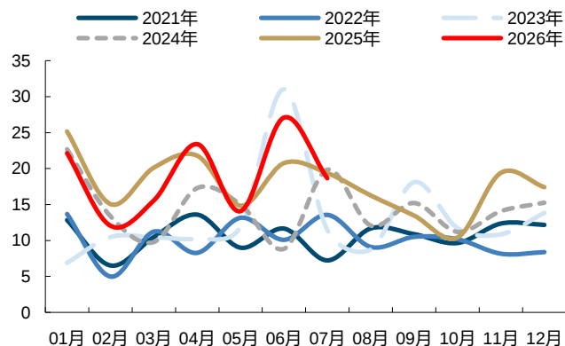
图表33：锆矿砂及其精矿进口量（万吨）
