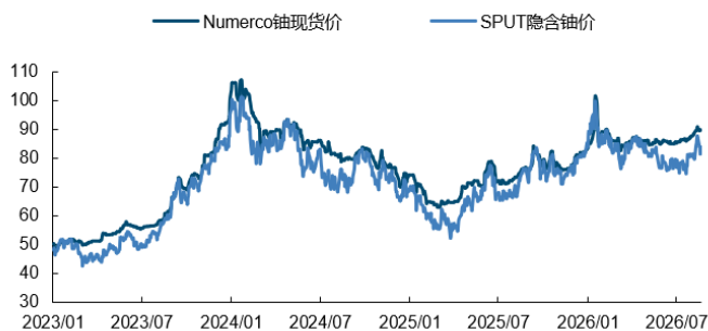
图表24: 铀日度现货价格及SPUT隐含价格 (美元/磅U3O8)
