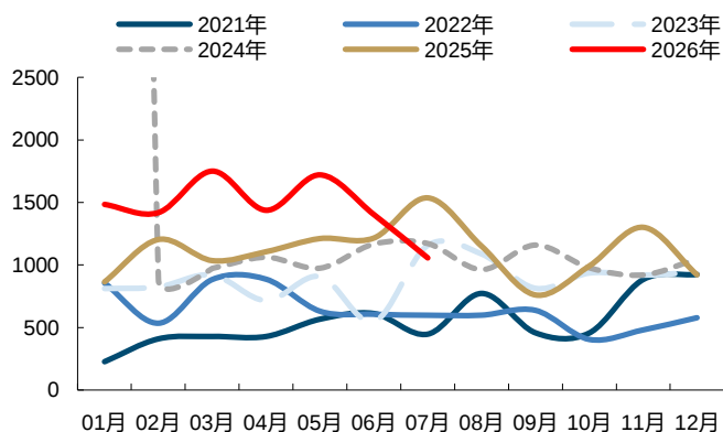
图表29：我国铌、钽、钒矿砂及其精矿进口量（吨）
