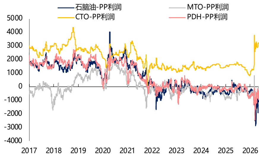
油煤气路线制聚丙烯盈利对比（元/吨）
