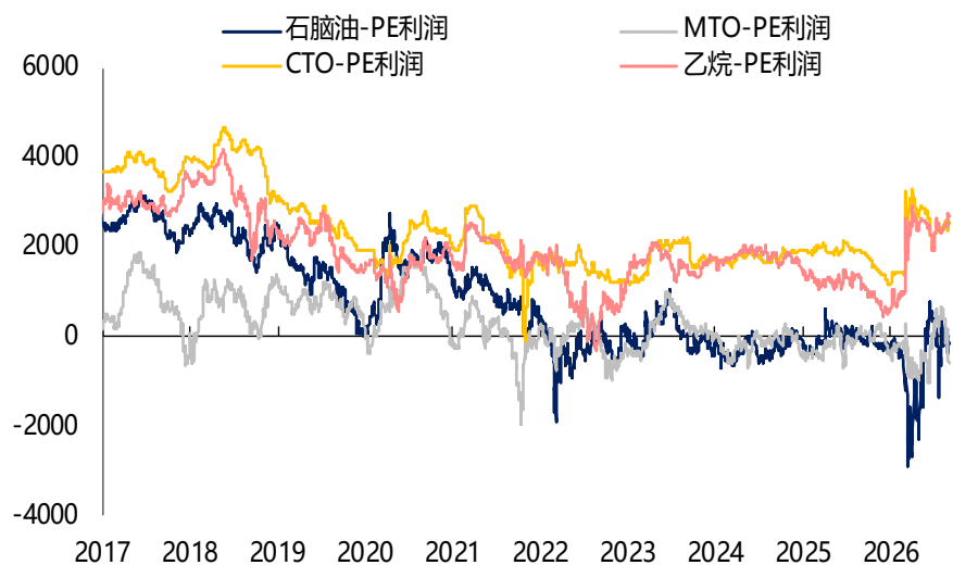
油煤气路线制聚乙烯盈利对比（元/吨）
