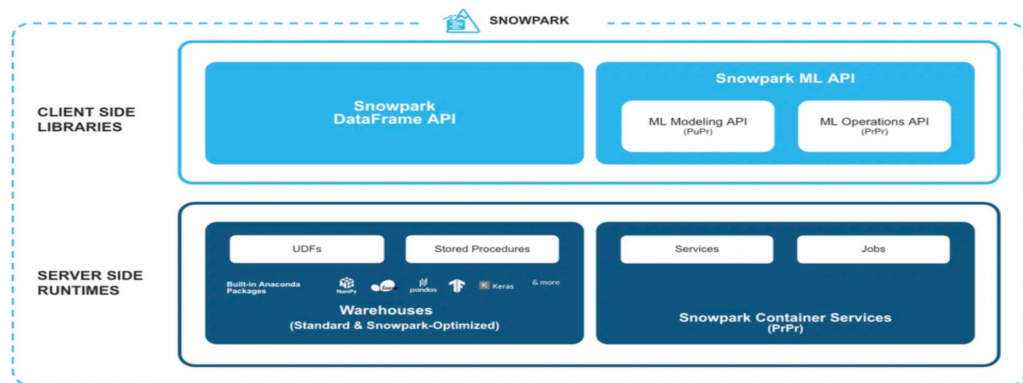
图：Snowpark 架构图
