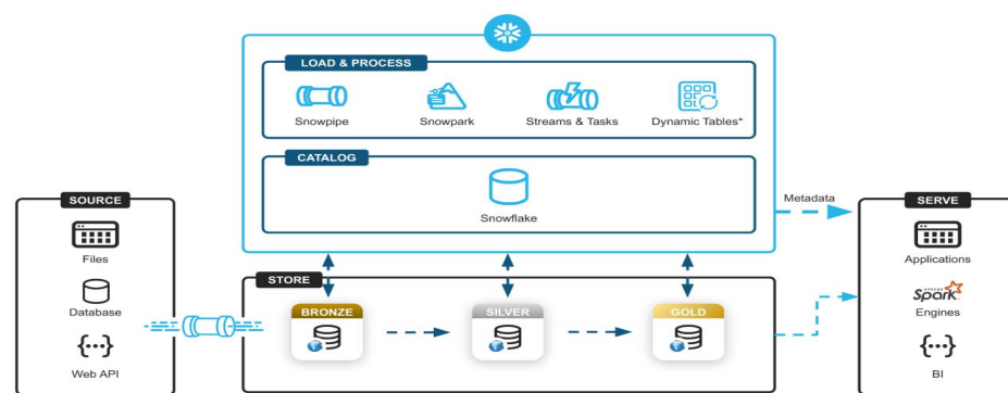
图：Snowflake Iceberg表交互架构
