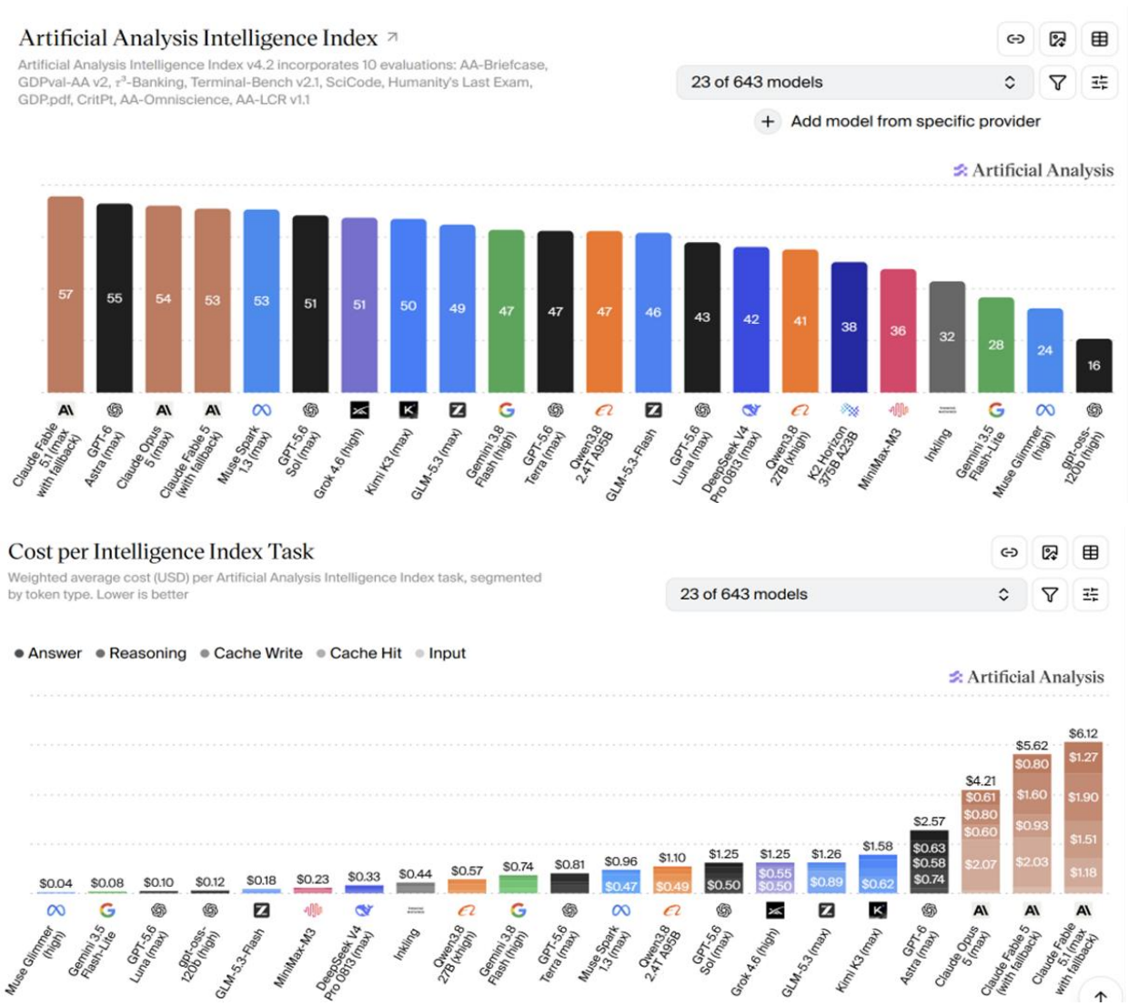
图 8：全球大模型人工智能指数及单任务成本
