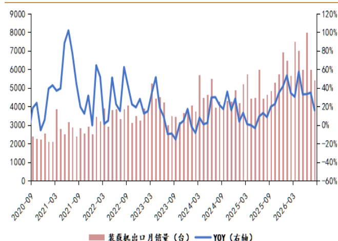
图 6：装载机外销台数和增速
