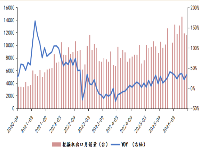
图 4: 挖机外销台数和增速
