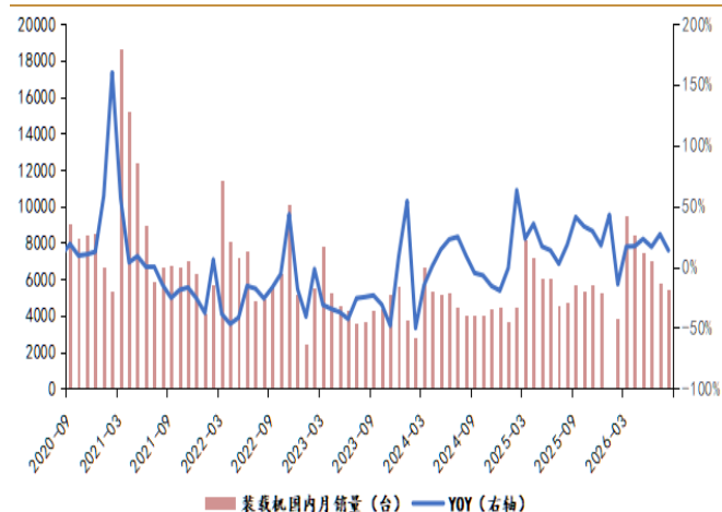
图 5：装载机内销台数和增速
