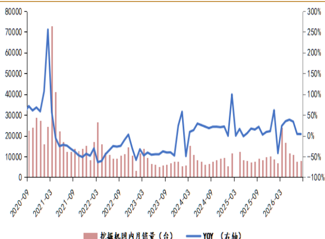
图 3: 挖机内销台数和增速
