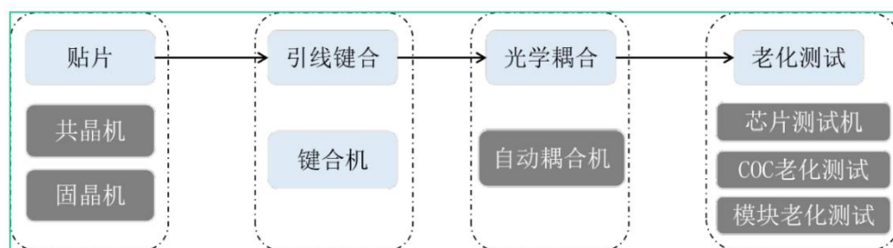
图 1：光模块生产封测各流程使用的主要设备
